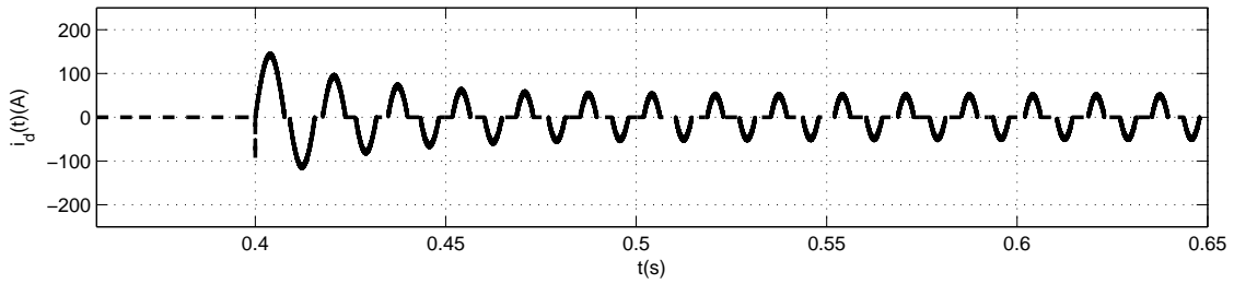
Figura 9: Simulação - \omega_{c1} = 1 .
