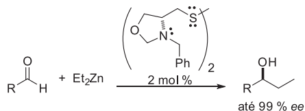
Esquema 4. Catalisador enantiopuro contendo enxofre para adição assimétrica de dietilzínco a aldeídos
