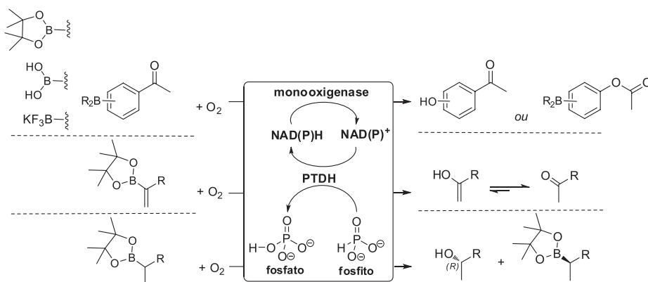
Esquema 3. Seletividade de reações de compostos de boro catalisadas por monooxigenases. PTDH = Fosfito desidrogenase
